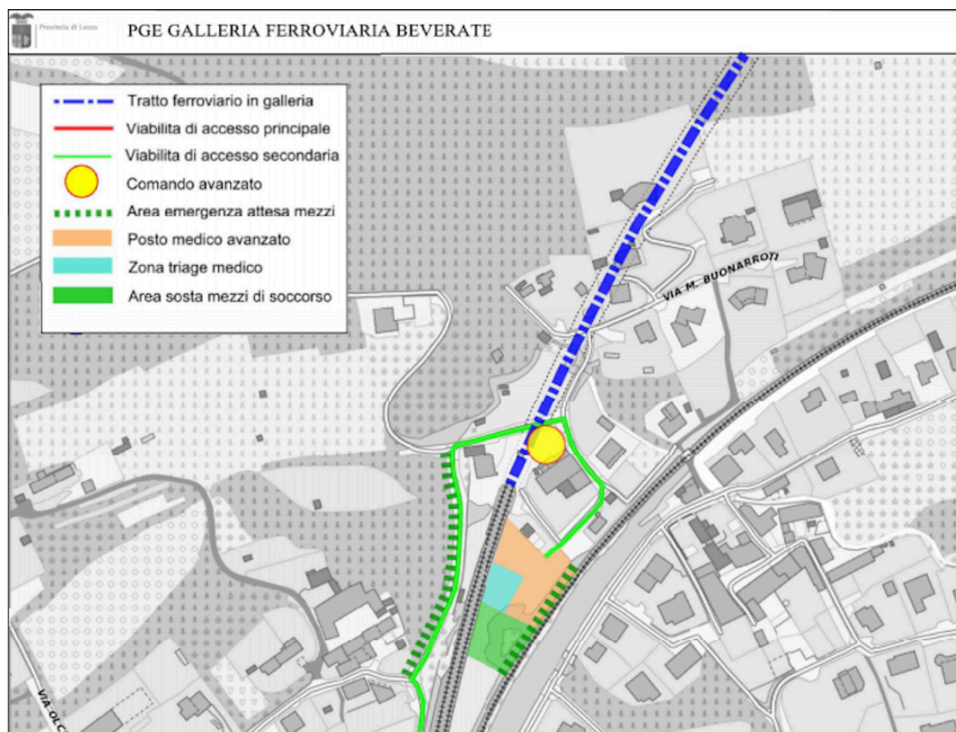
Una tavola del piano di gestione emergenziale della Galleria Beverate
